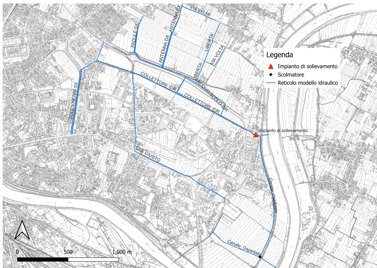
Figura 2-2 – Schema configurazione 1.
