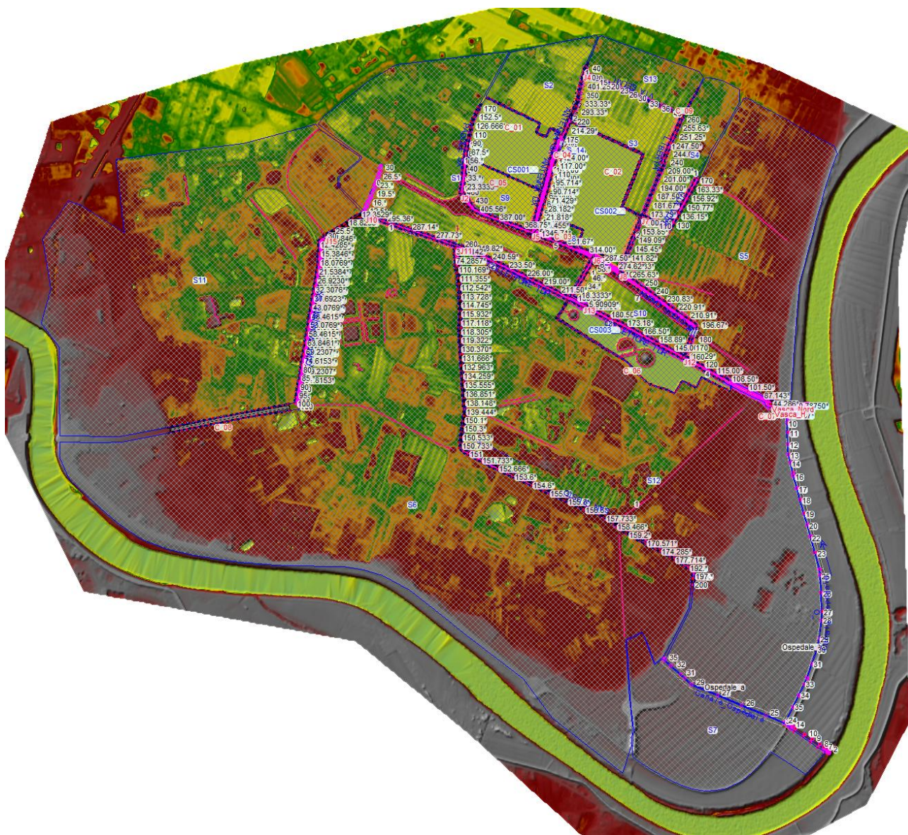
Figura 4-2 – Estratto modello idraulico
