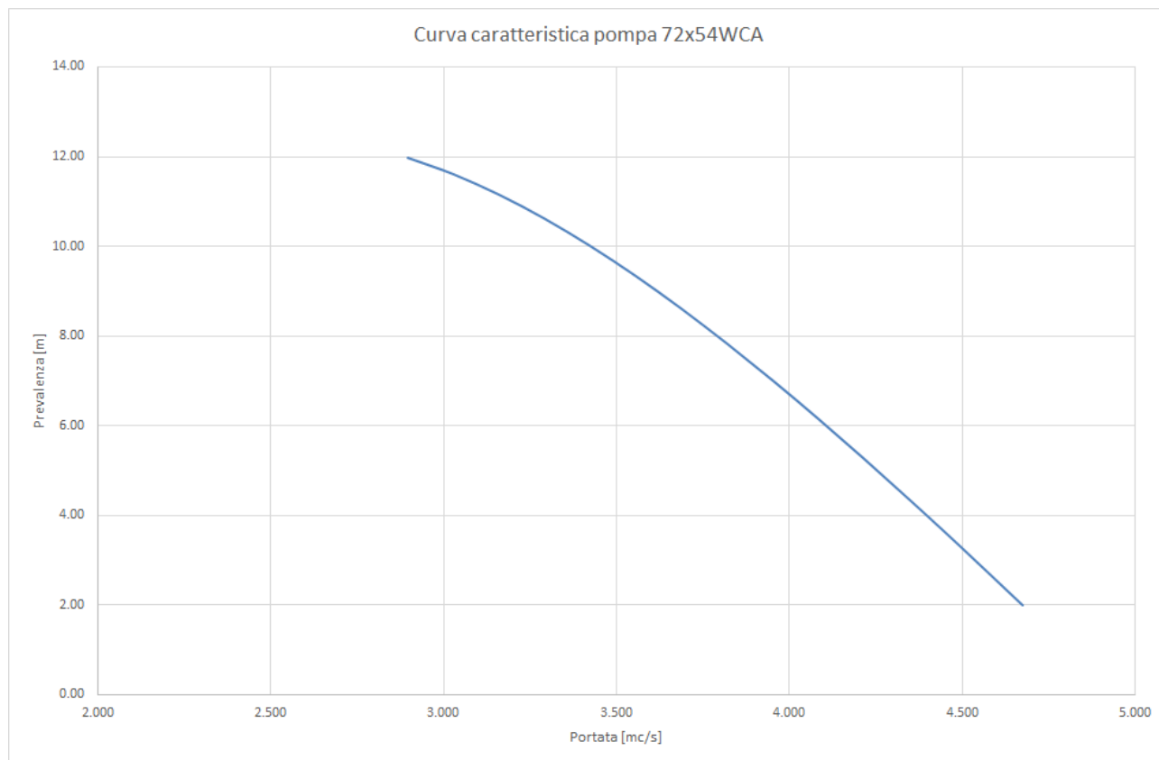
Figura 2-3 – Curva caratteristica pompa principale.
